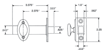
0419.xxx – 2.375" Backset Mortise Bolt
